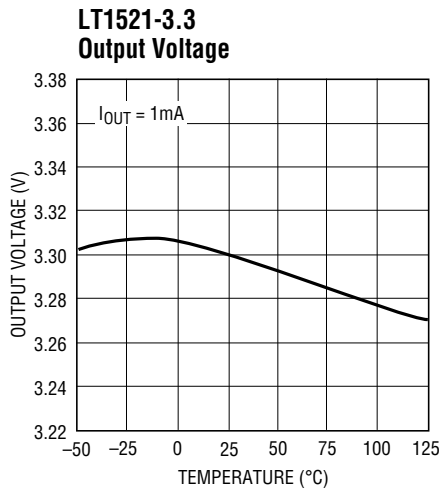
LT1521 • TPC05
