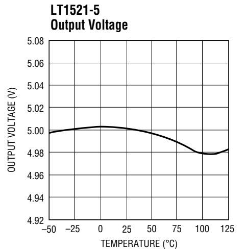
LT1521 • TPC06
