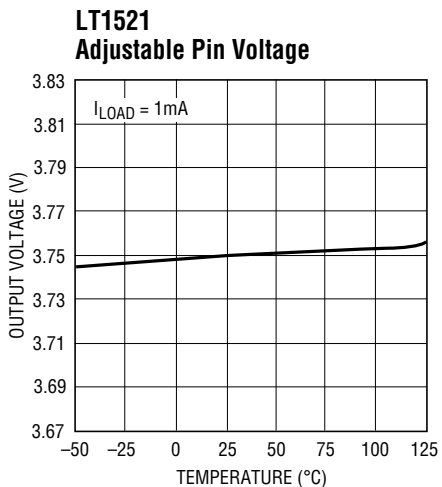
LT1521 • TPC07
