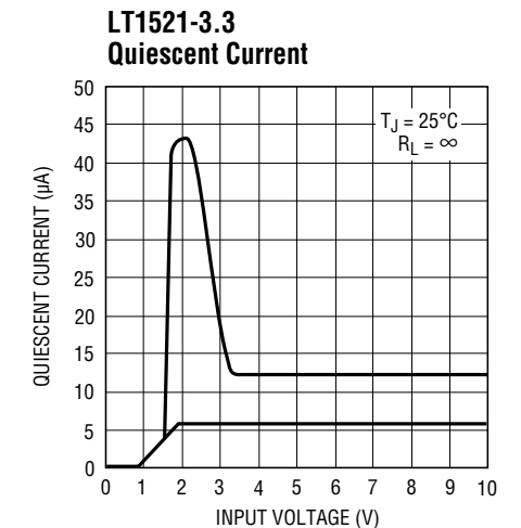
LT1521 • TPC09
