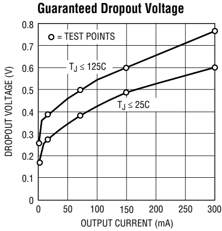
LT1521 • TPC01
