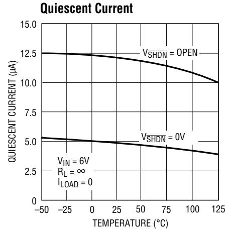
LT1521 • TPC03
