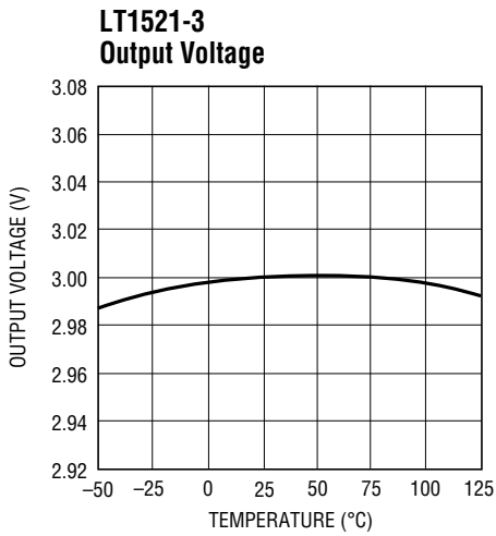
LT1521 • TPC04
