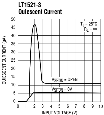
LT1521 • TPC08
